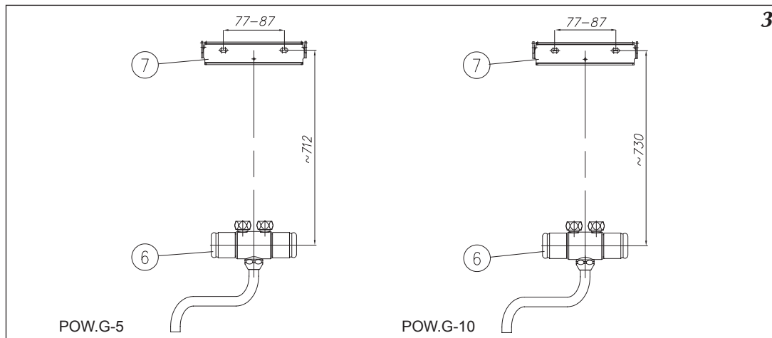
Рис.3 Монтаж водонагревателя POW.G на вешалке
