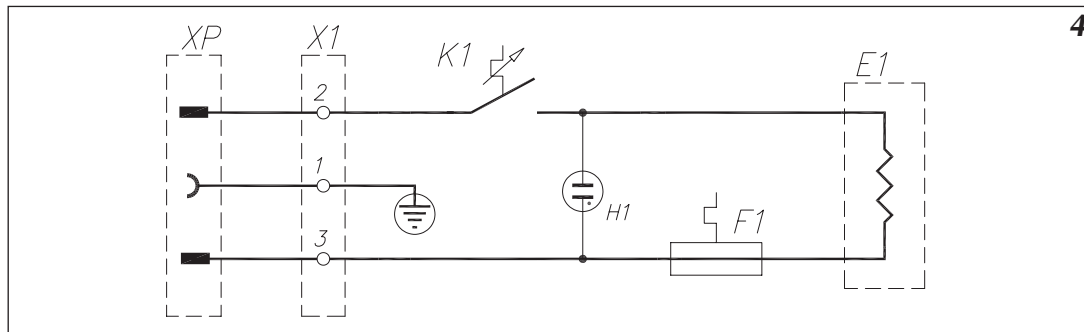
Рис.4 Принципиальная схема
